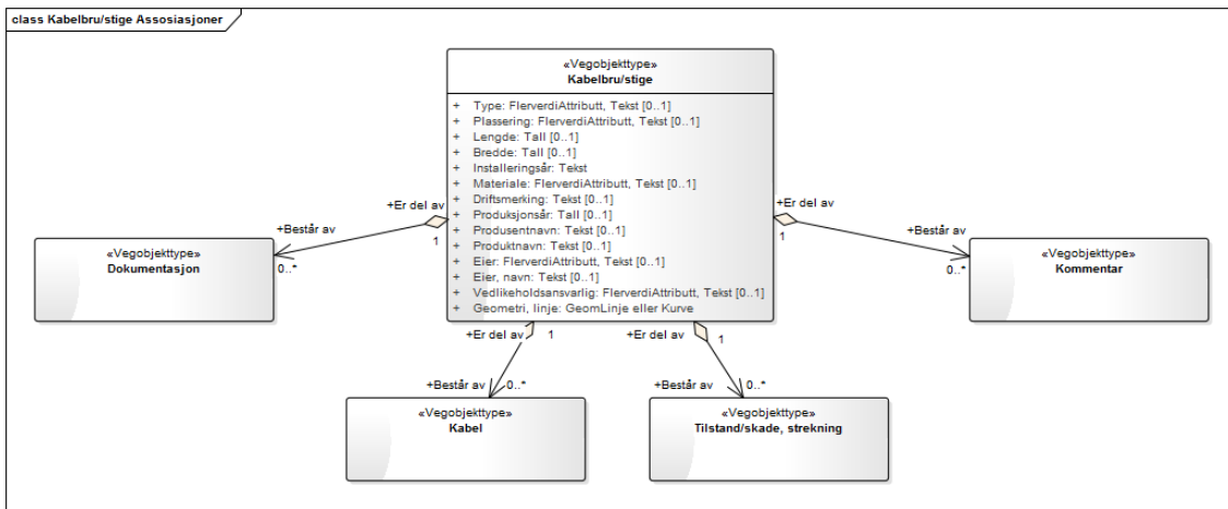
Figur 2: UML-modell for Kabelbru/stige med assosiasjoner
