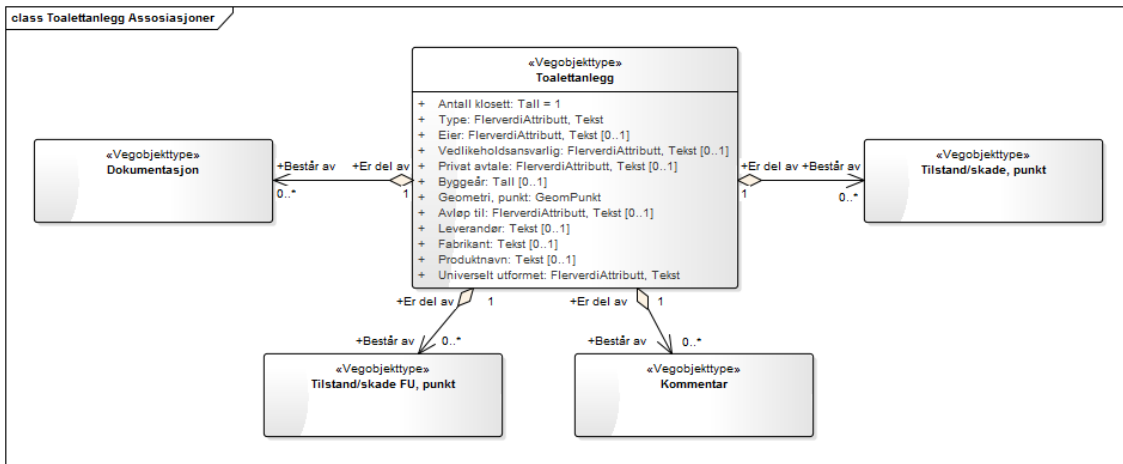
Figur 2: UML-skjema Toalettanlegg med assosiasjoner
