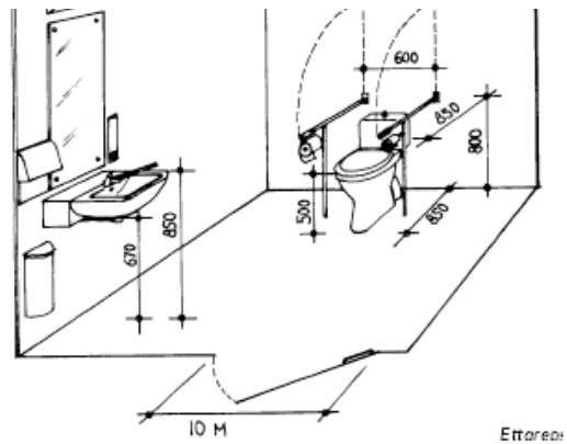
Figuren viser toalett med anbefalte mål for universell utforming
