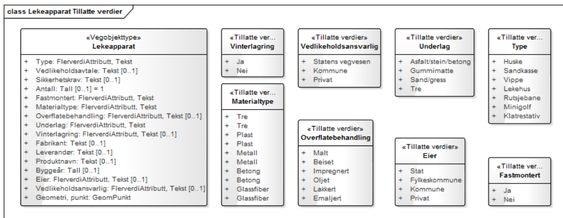
Figur 1: UML-skjema Lekeapparat
