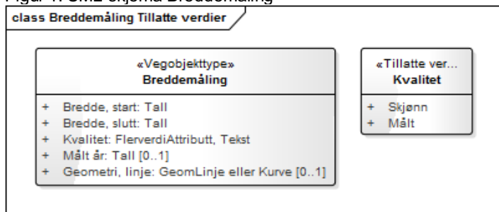
Figur 1: UML-skjema Breddemåling
