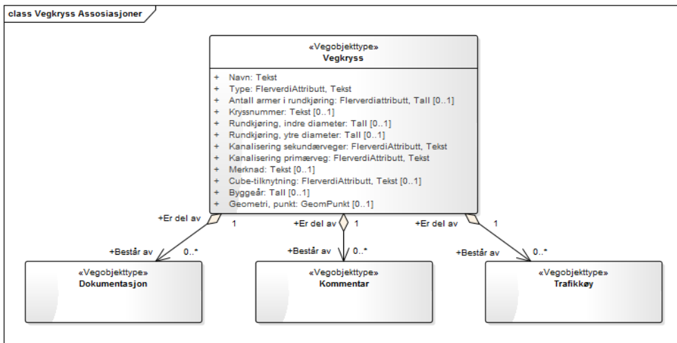
Figur 2: UML-skjema Vegkryss med assosiasjoner
