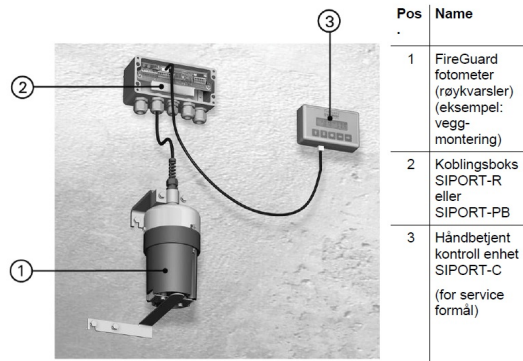
Figur 3: Brann-detektor for tunnel. Foto: SIGRIST
