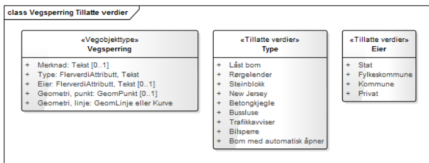
Figur 1: UML-skjema Vegsperring
