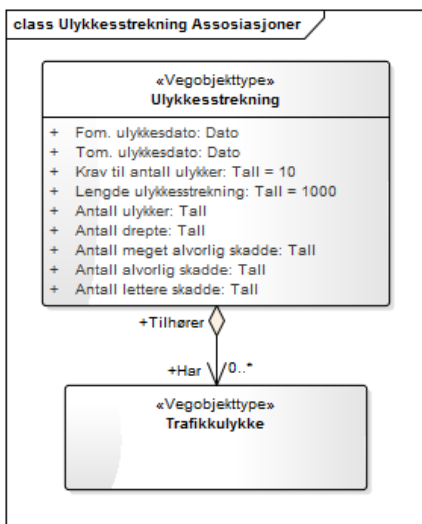
Figur 2: UML-skjema med assosiasjoner for ulykkesstrekning
