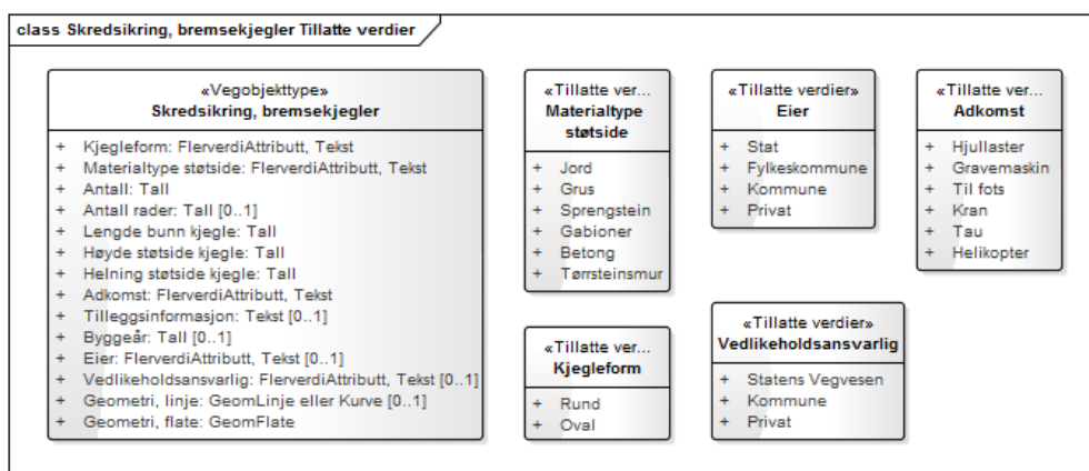
Figur 1: UML-skjema for Skredsikring, bremsekjegler
