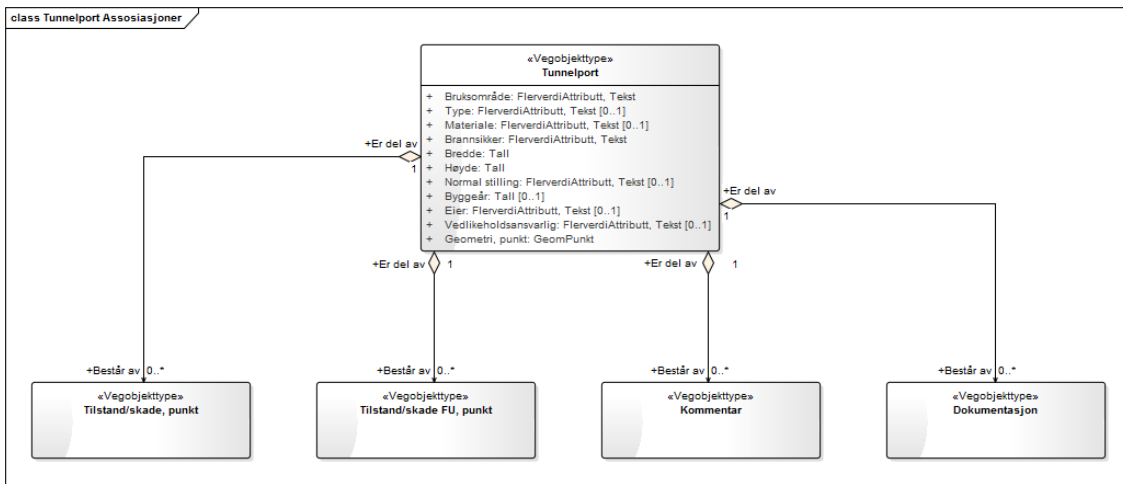
UML-skjema for Tunnelport med assosiasjoner
