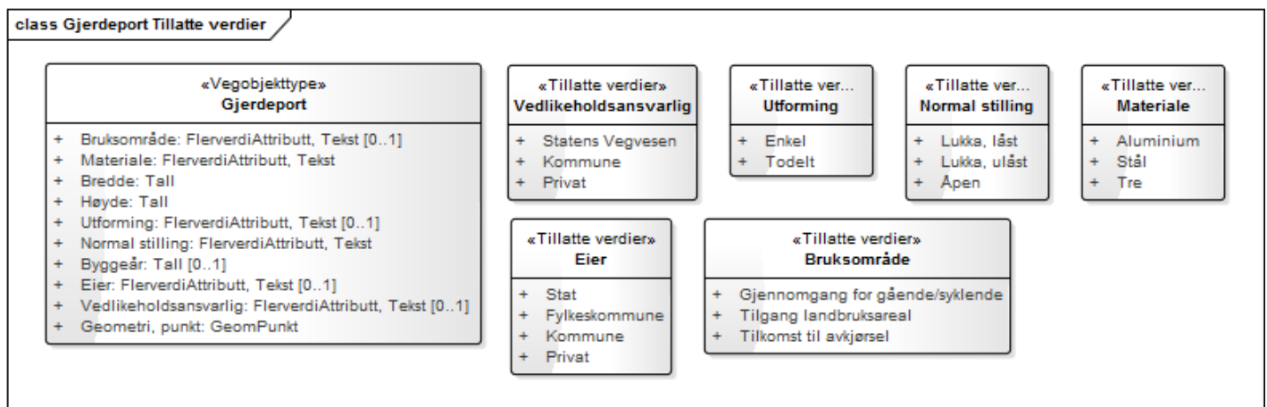
Figur 1: UML-skjema for Gjerdeport
