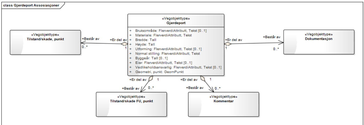
UML-skjema for Gjerdeport med assosiasjoner
