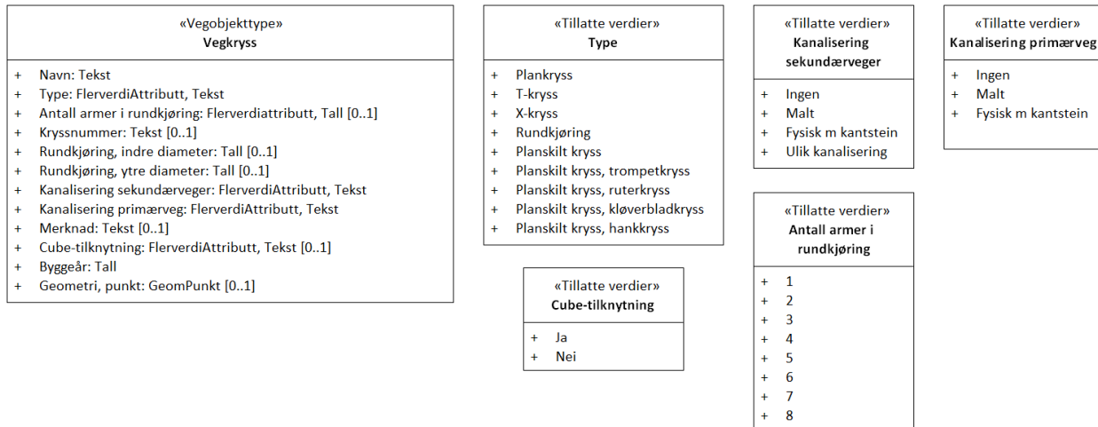
Figur 2:UML-skjema tillatte verdier
