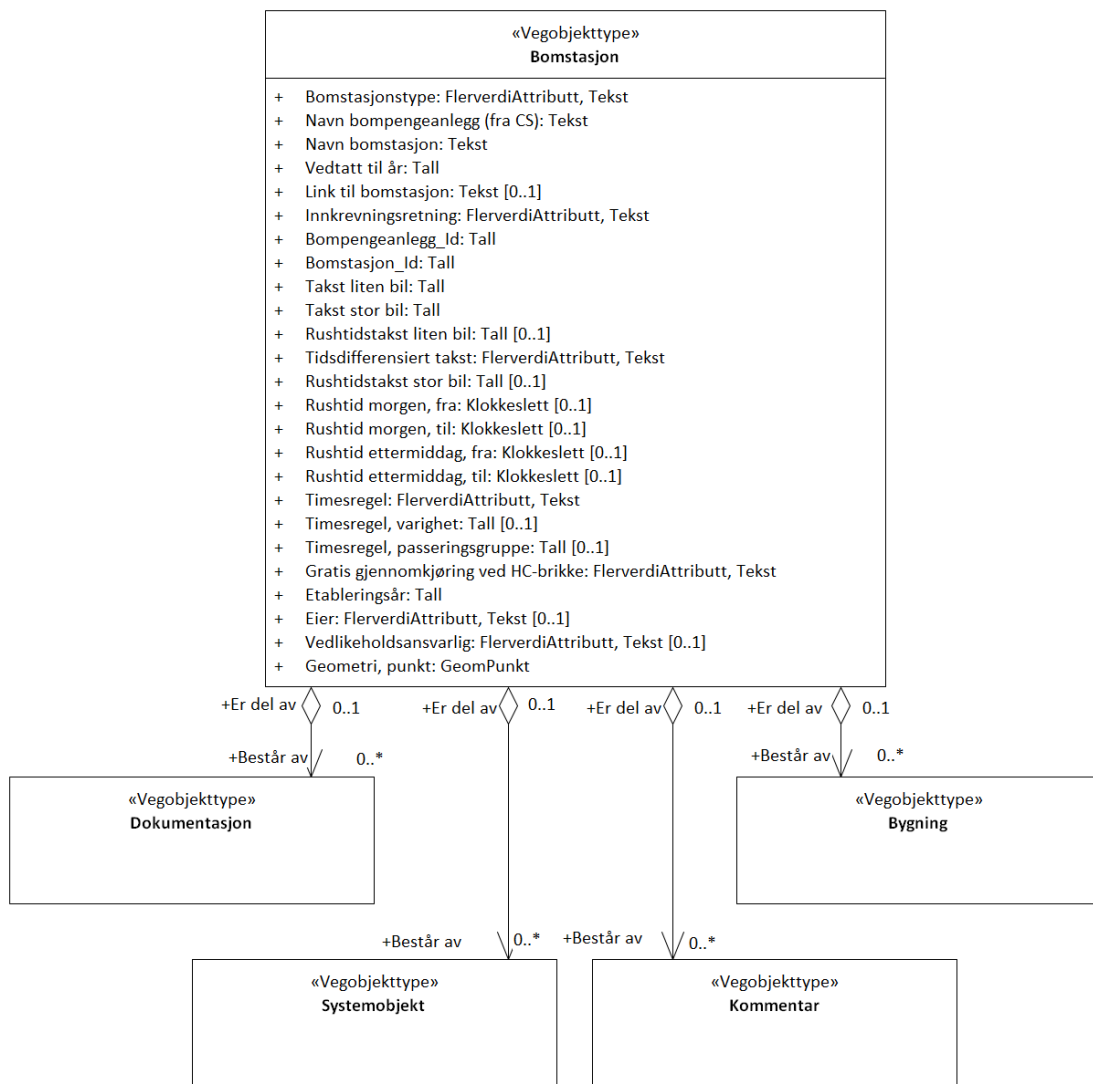
Figur 3: UML-skjema med assosiasjoner
