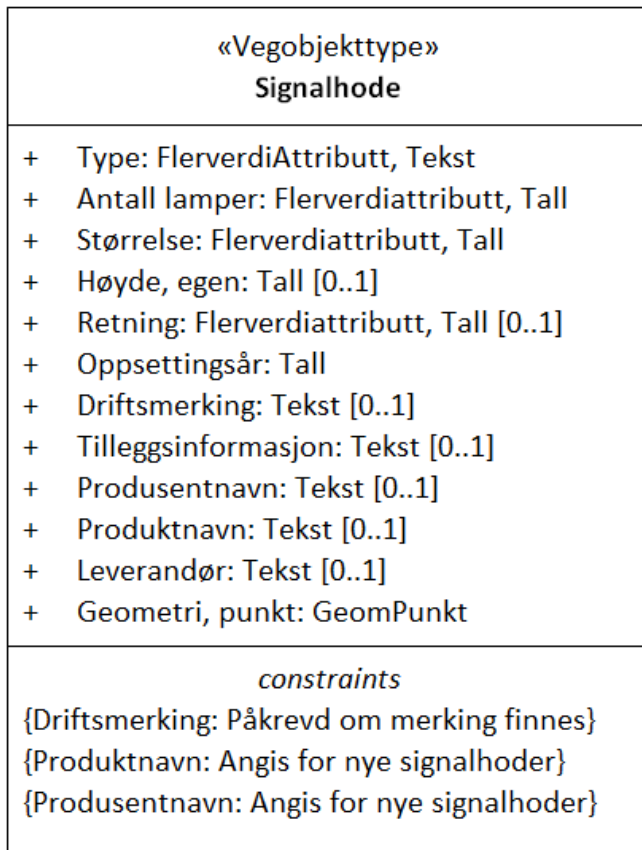
Figur 1: UML-skjema Signalhode
