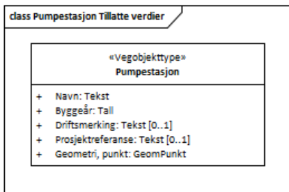
Figur 2: UML-skjema tillatte verdier
