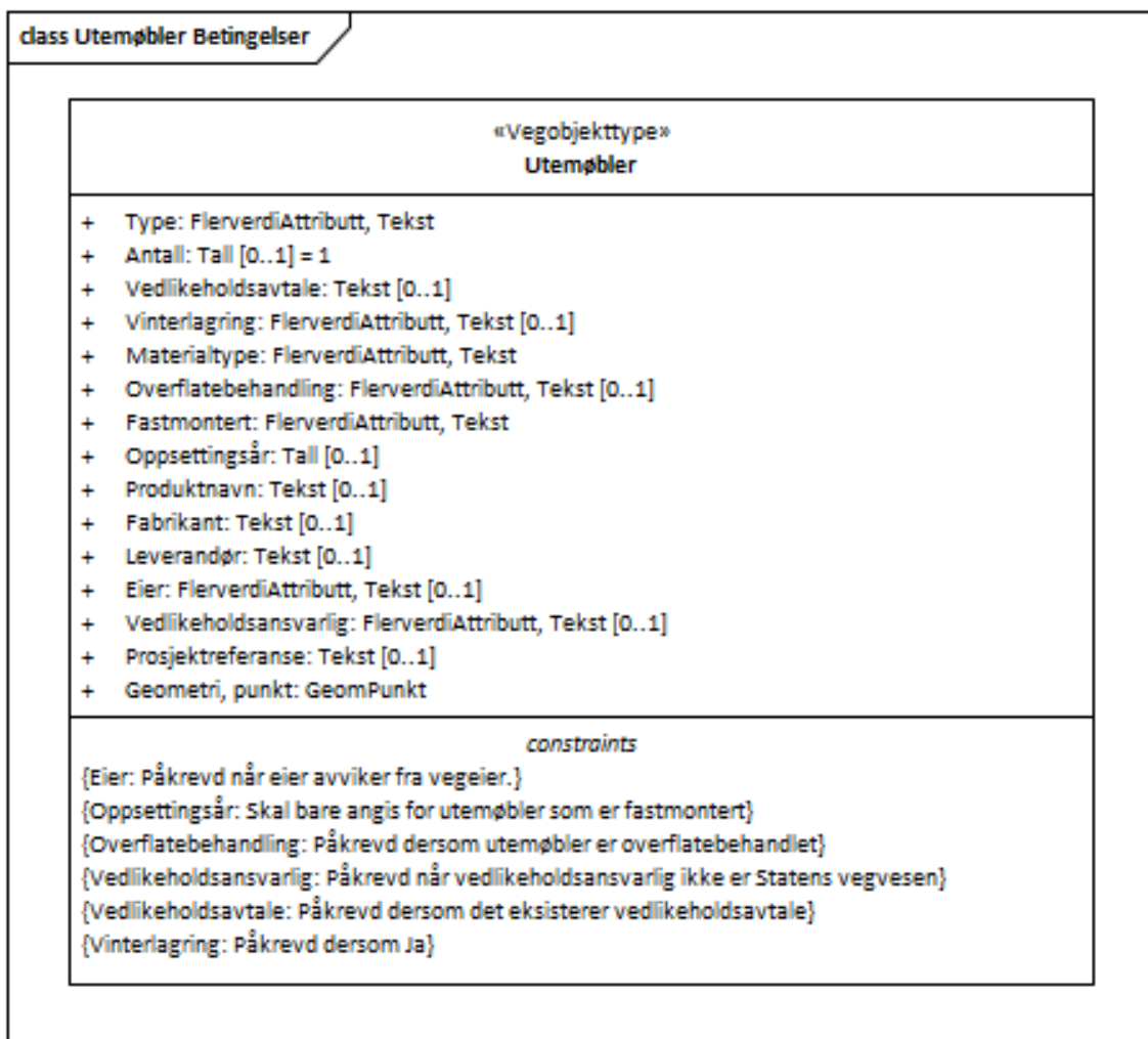
Figur 1: UML-skjema Utemøbler
