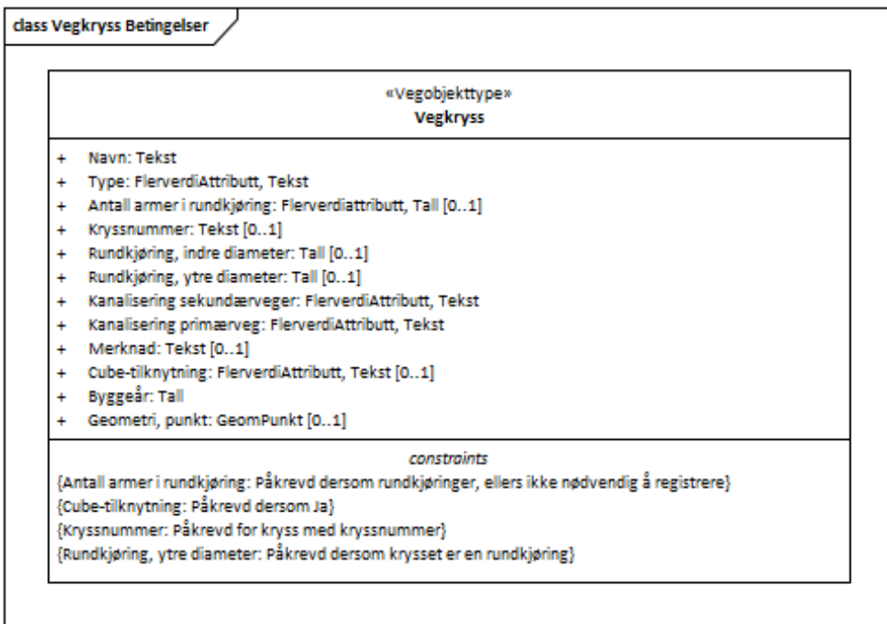
Figur 1:UML-skjema Vegkryss
