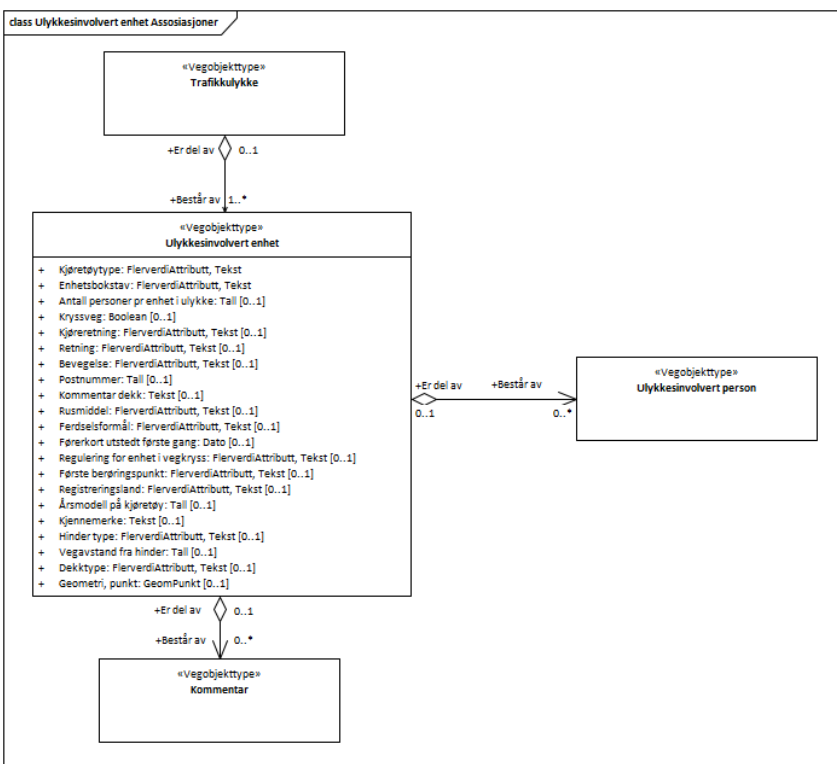
Figur 3: UML-skjema med assosiasjoner
