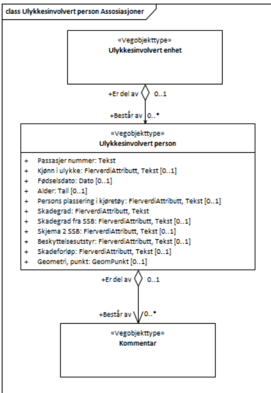
Figur 3: UML-skjema med assosiasjoner
