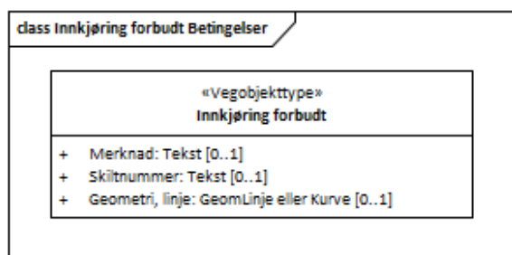
Figur 1: UML-skjema
