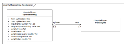
Figur 3: UML-skjema med assosiasjoner
