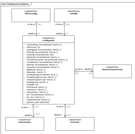
Figur 3: UML-skjema med assosiasjoner
