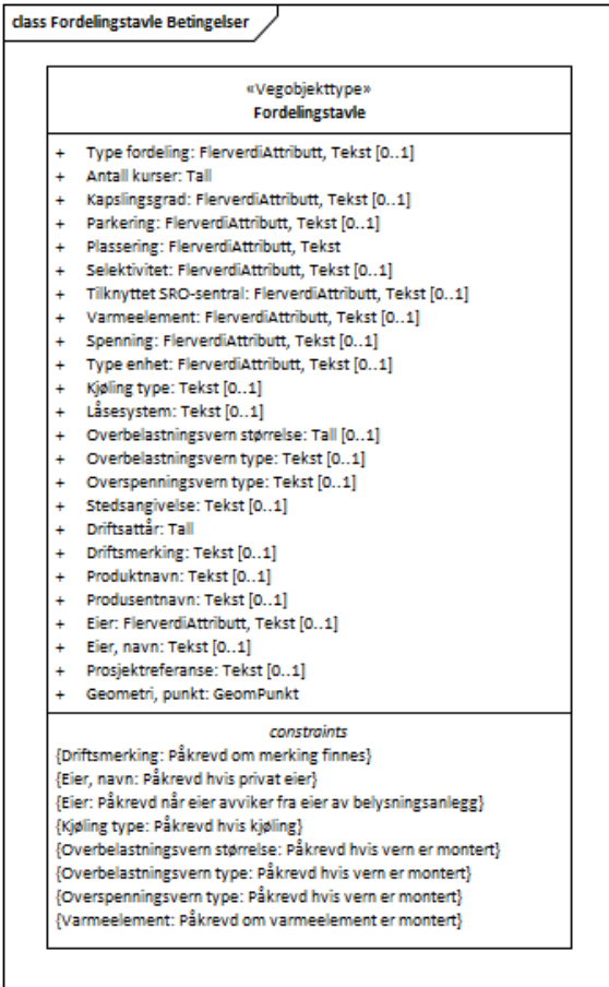
Figur 1:UML-skjema med betingelser
