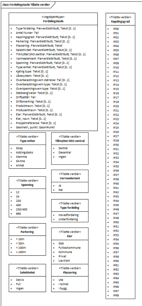
Figur 2: UML-skjema tillatte verdier
