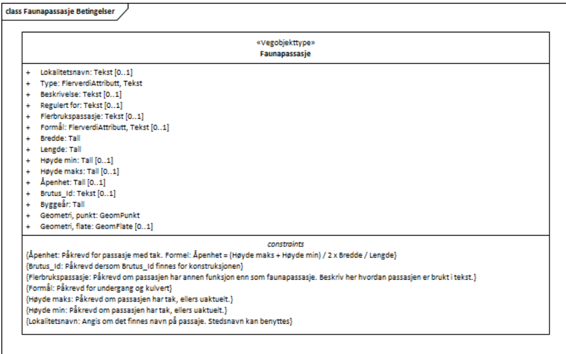
Figur 1: UML-skjema med betingelser
