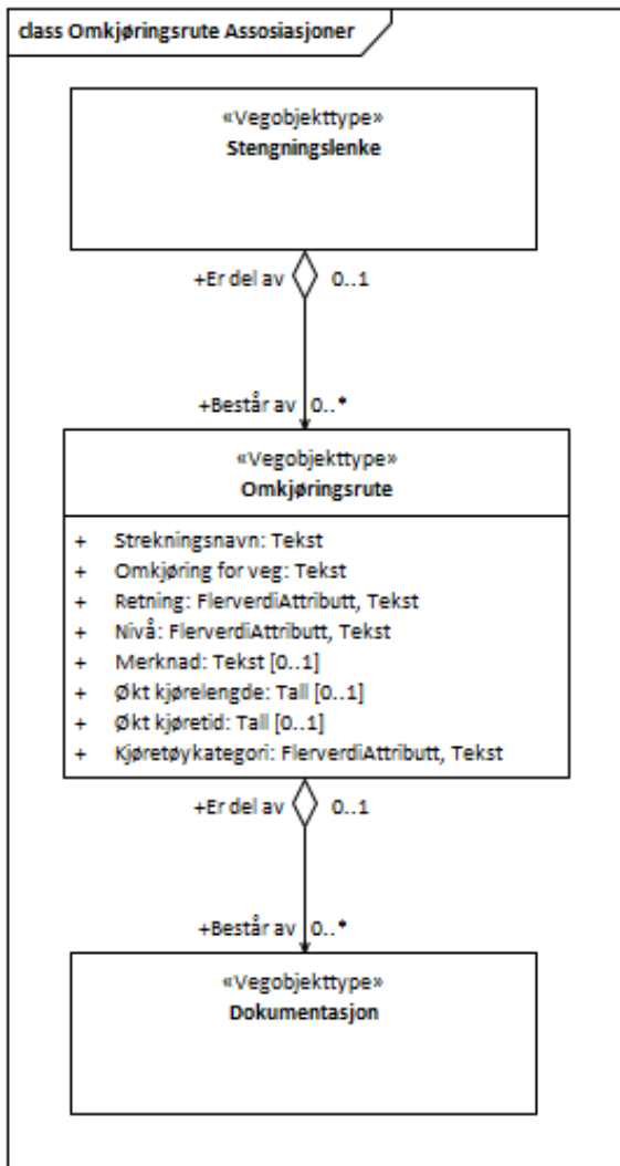
Figur 3: UML-skjema med assosiasjoner
