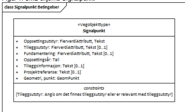
Figur 1: UML-skjema Signalpunkt
