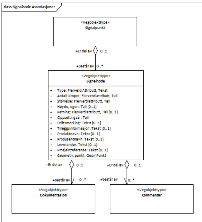
Figur 3: Assosiasjoner
