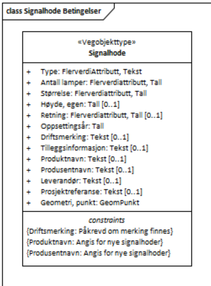
Figur 1: UML-skjema Signalhode
