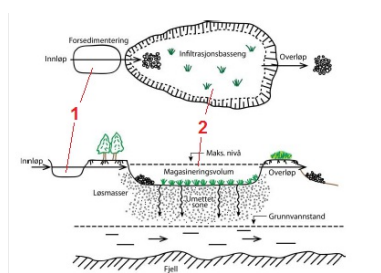
Figur 403.4. Utforming av infiltrasjonsbasseng (plan/snitt)
