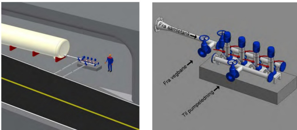
Rorteknisk illustrasjon i en typisk trinnpumpestasjon. Til venstre: samletank med pumper. Til høyre: detalj av vannvei for pumpevann i et pumpetrinn.
