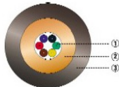
TBW LSZH Fiberkabel
