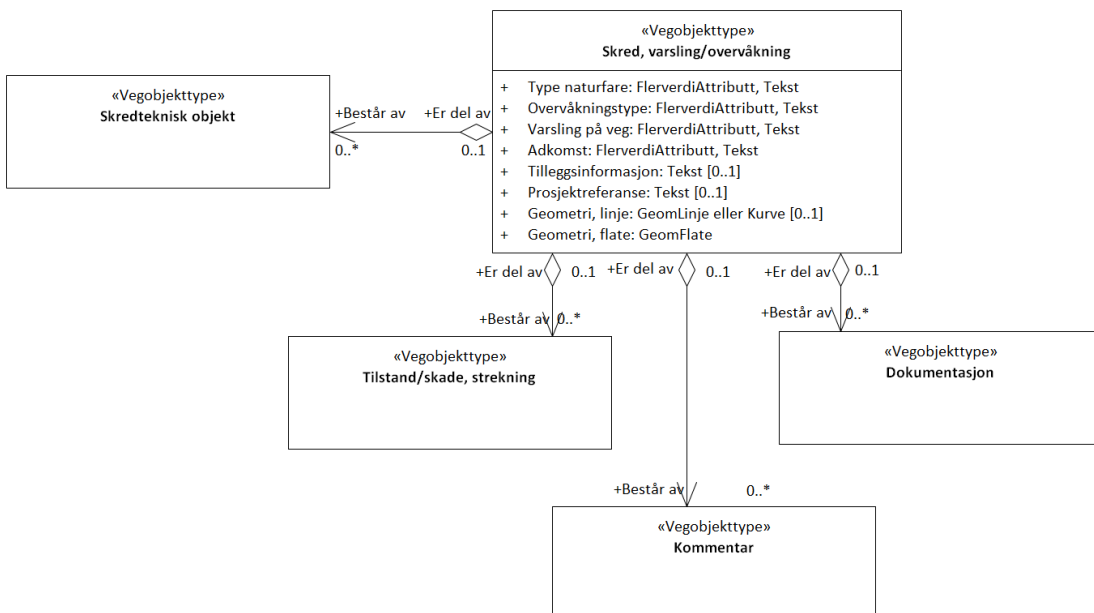
Figur 3: UML-skjema med assosiasjoner
