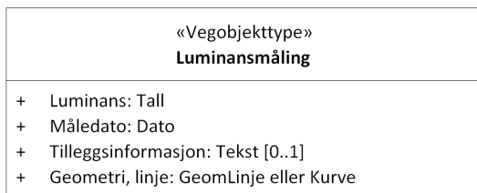
Figur 2: UML-skjema tillatte verdier
