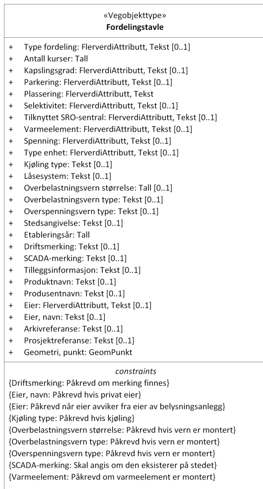
Figur 1:UML-skjema med betingelser
