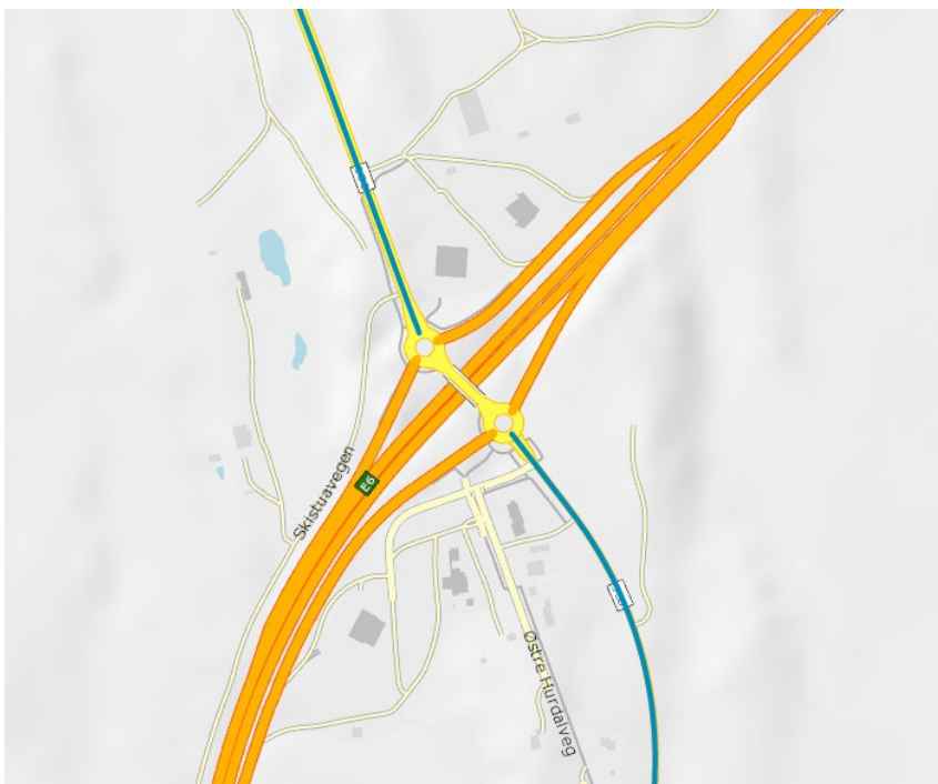
Figur 9: Startpunkt for omkjøringsruter (blå) starter nedstrøms rundkjøringar når de representerer forgreiningar inn mot hovedvegen med stengningsløyen (ikke vist her).
