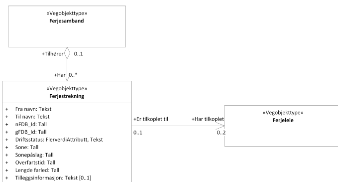
Figur 3: UML-skjema med assosiasjoner
