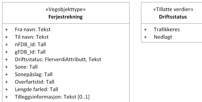
Figur 2: UML-skjema tillatte verdier
