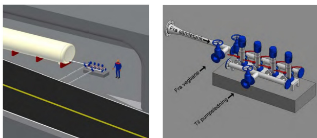
Rørteknisk illustrasjon i en typisk trinnpumpestasjon. Til venstre: samletank med pumper. Til høyre: detalj av vannvei for pumpevann i et pumpetrinn.
