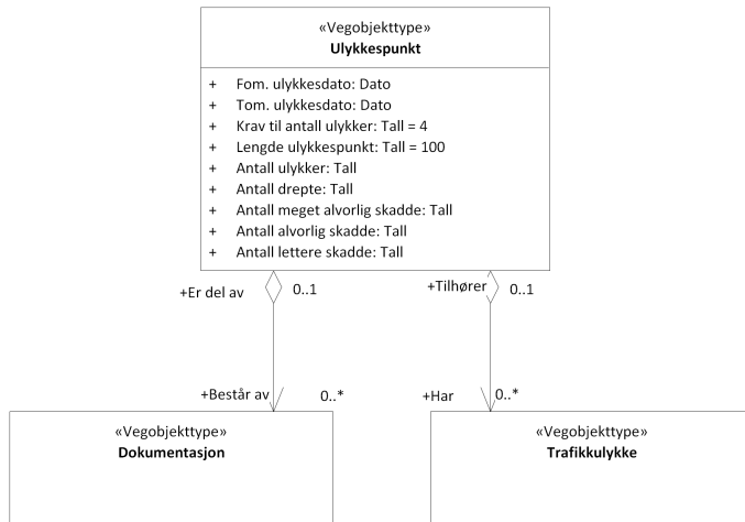
Figur 3: UML-skjema med assosiasjoner
