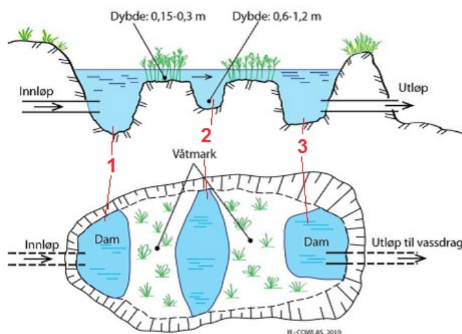
Figur 403.8. Prinsippskisse av kunstig anlagt våtmark (plan/snitt).
