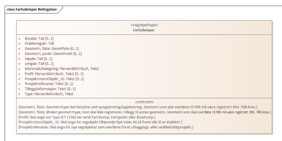
Figur 1: UML-skjema med betingelser
