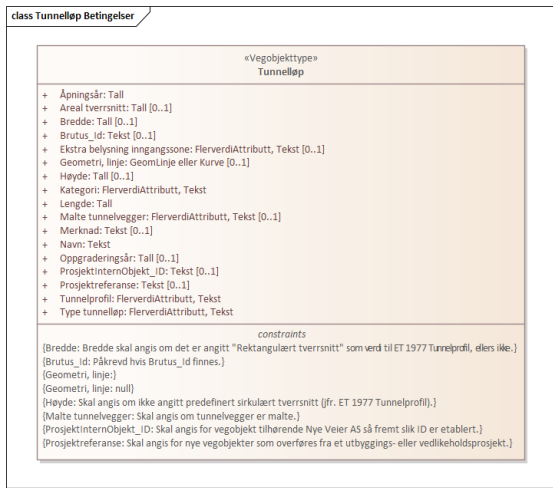
Figur 1: UML-skjema Tunneløp
