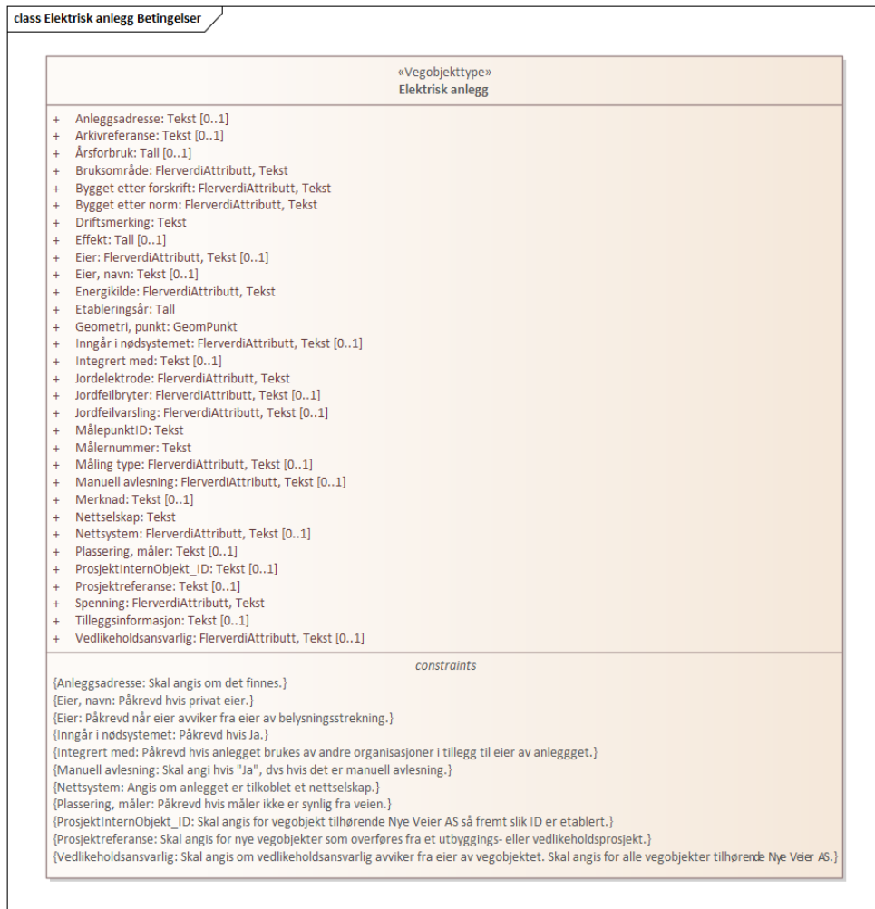
Figur 1: UML-skjema med betingelser
