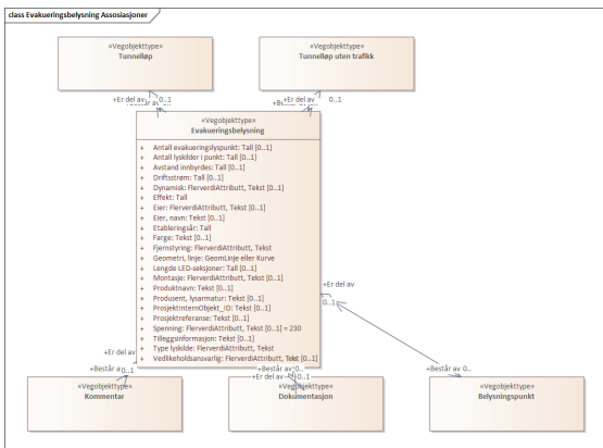
Figur 3: UML-skjema med assosiasjoner
