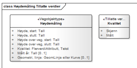
Figur 1: UML-skjema Høydemåling
