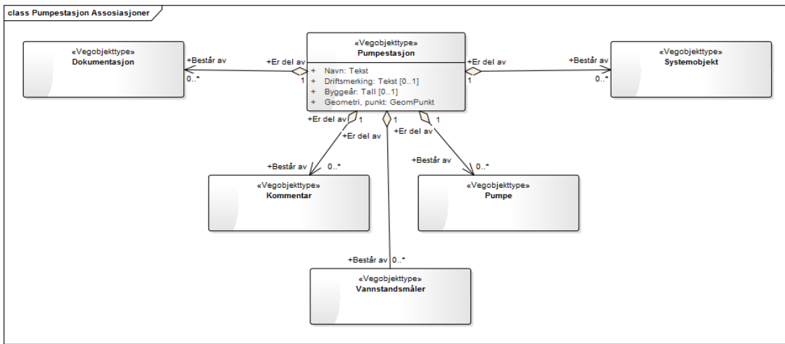
UML-skjema for Pumpestasjon med assosiasjoner
