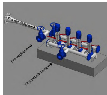
Rørteknisk illustrasjon i en typisk trinnpumpe-stasjon. Til venstre: samletank med pumper. Til høyre: detalj av vannvei for pumpevann i et pumpetrinn.
