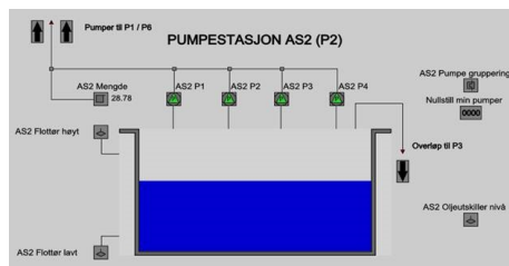
Skjema for pumpestasjon fra Vegvokteren
