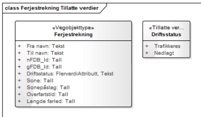
Figur 1: UML-skjema for Ferjestrekning
