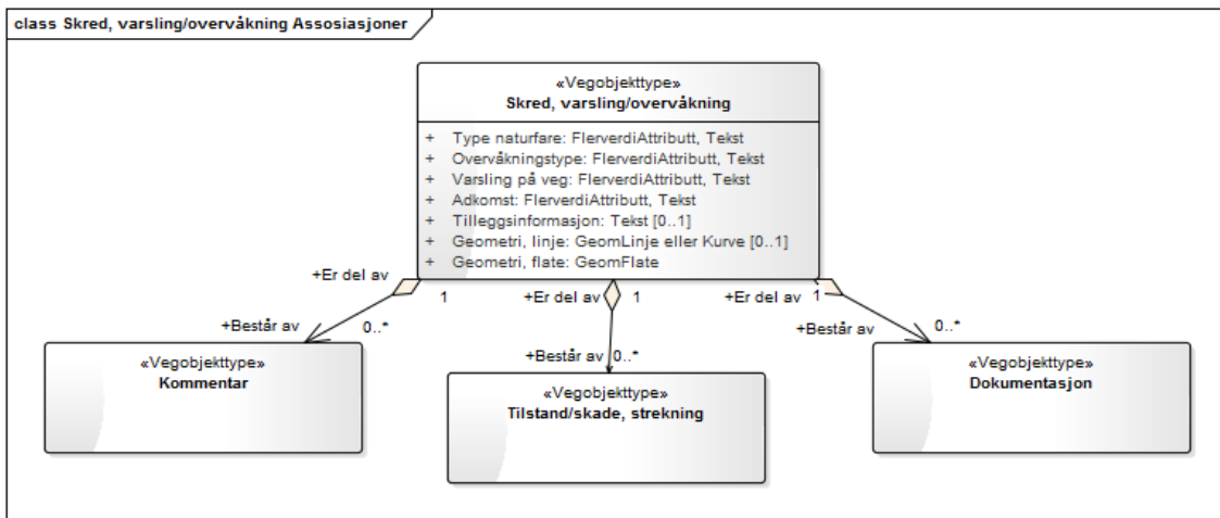
Figur 2: UML-skjema for Skred, varsling/overvåkning med assosiasjoner
