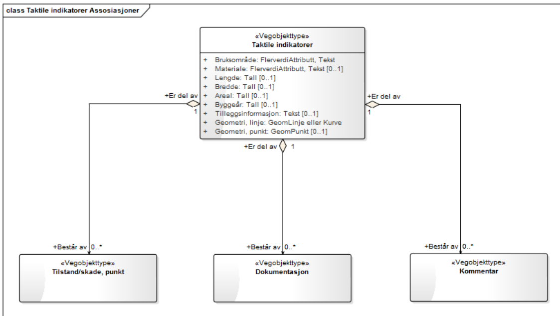
Figur 2: UML-skjema for Taktile indikatorer med assosiasjoner
