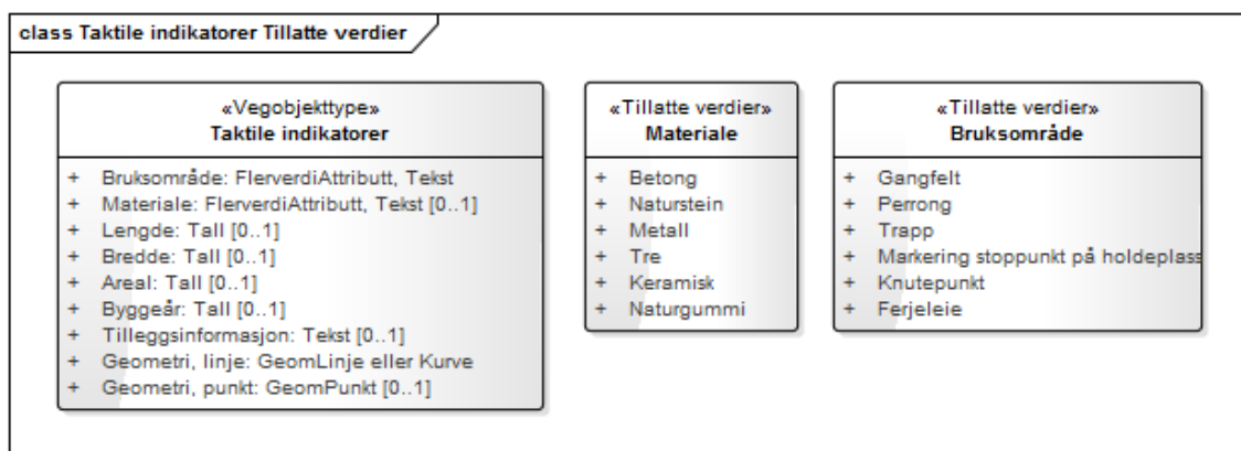
Figur 1: UML-skjema for Taktile indikatorer
