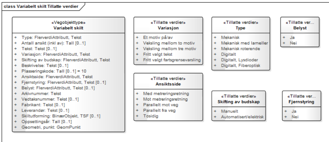
Figur 1: UML-skjema Variabelt skilt
