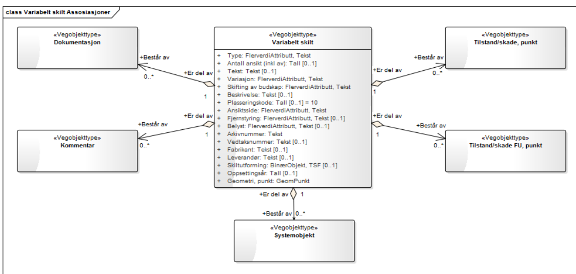
Figur 2: UML-skjema Variabelt skilt
