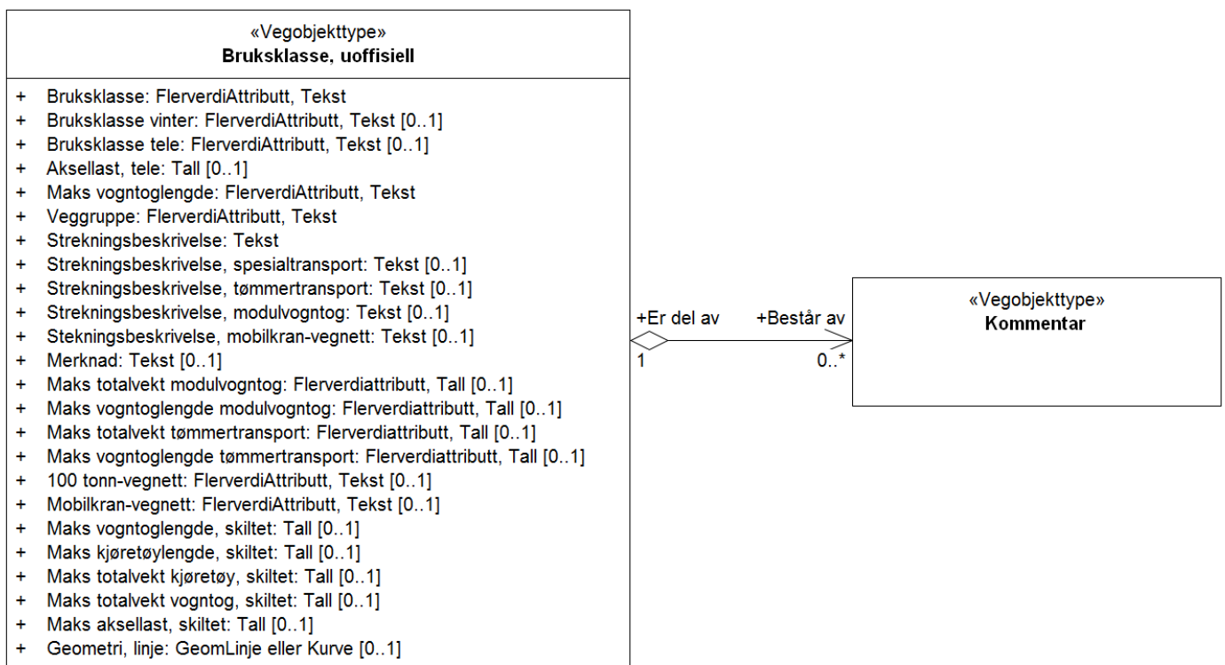
Figur 3: UML-skjema med assosiasjoner
