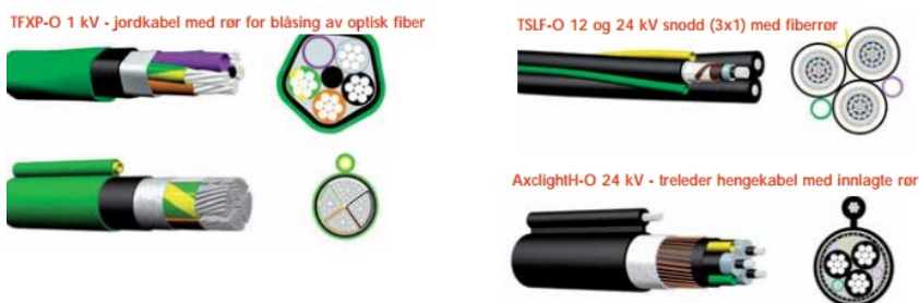
Figur 5: Kraftkabel med innlagt fiberrør
