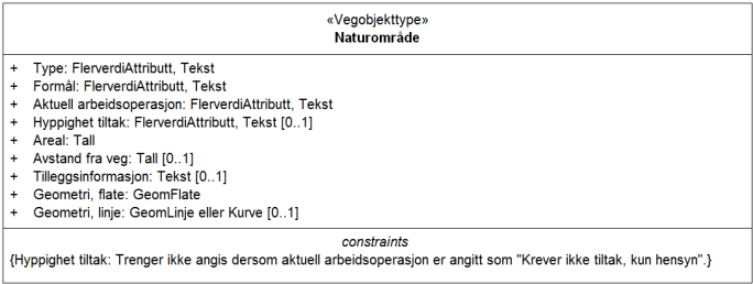
Figur 1: UML-skjema med betingelser
