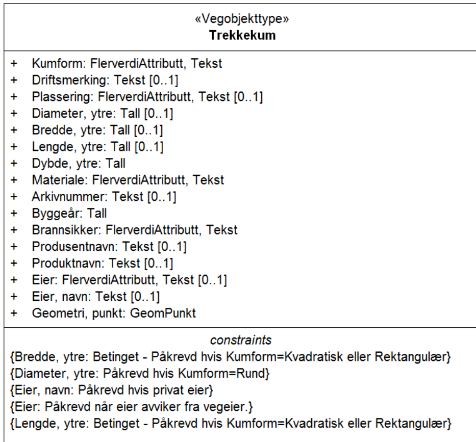
Figur 1: UML-skjema for Trekkefum
